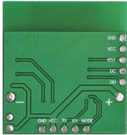
(模块背面图)
